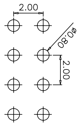
P.C.B LAYOUT
