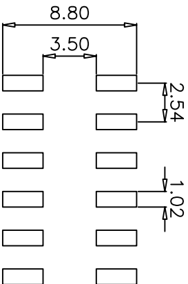
P.C.B LAYOUT
