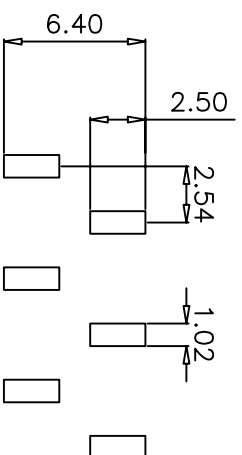
P.C.B LAYOUT
