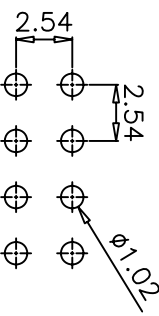
P.C.B LAYOUT
