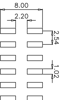
P.C.B LAYOUT
