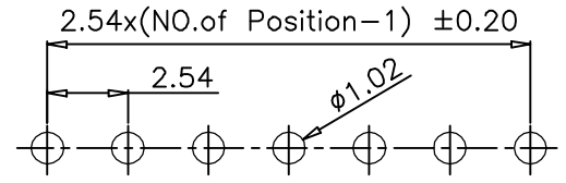
P.C.B LAYOUT
