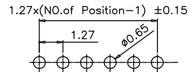
P.C.B LAYOUT
